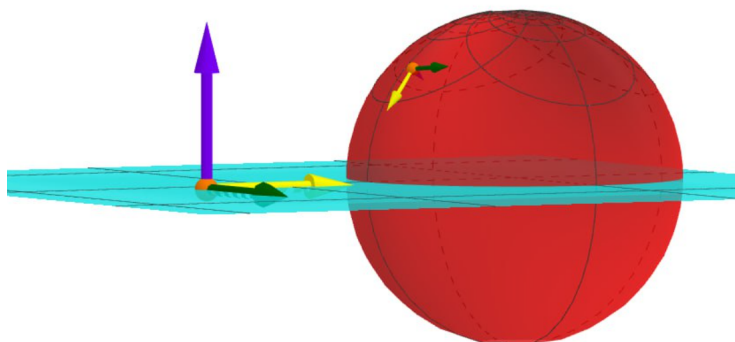
Figura 2.6: Orientació des de fora de \mathbb{S} .
