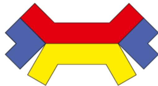
gran rombicuboctàedre
