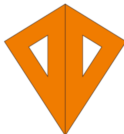
triacontàedre disdakís
