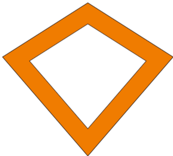
icositetràedre deltoïdal
