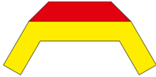
octàedre escapçat
