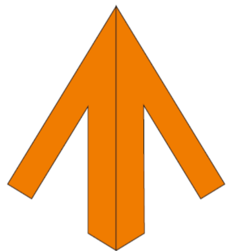
octàedre tetrakis
