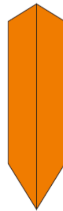
triacontàedre ròmbic
