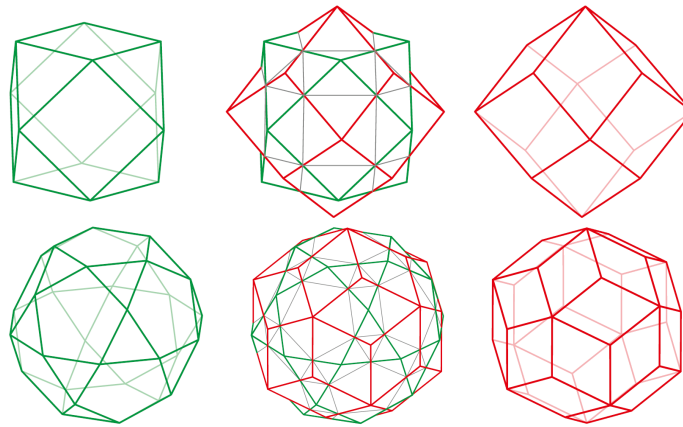
Figura 5: Primera fila: dualitat cuboctàedre – dodecàedre ròmbic. Segona fila: dualitat icosidodecàedre – triacontàedre ròmbic (el prefix grec triaconta significa trenta).
