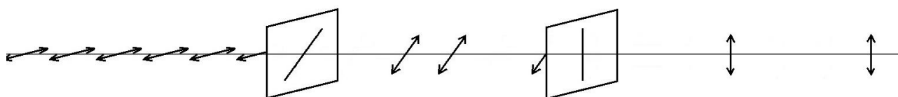
Fig. 2.6.2.2.5. Esquema on es mostra llum polaritzada horitzontalment passant per un polaritzador amb un angle de \pi/4 rad i seguidament per un de vertical. Passa un quart dels fotons, aproximadament.
