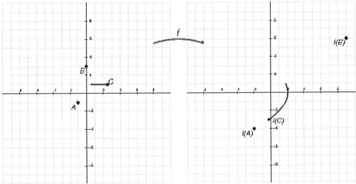
Gràfica en variable complexa
