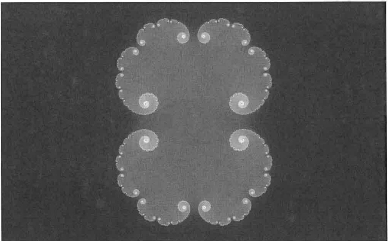
Conjunt de Julia f(z) = z^2 + 0.285
