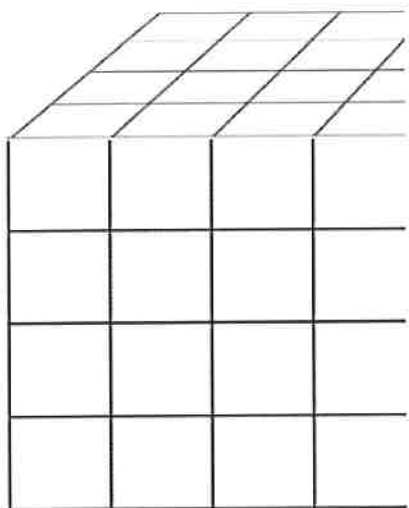
Cub de dimensió 3 dividit entre 64 trossos
