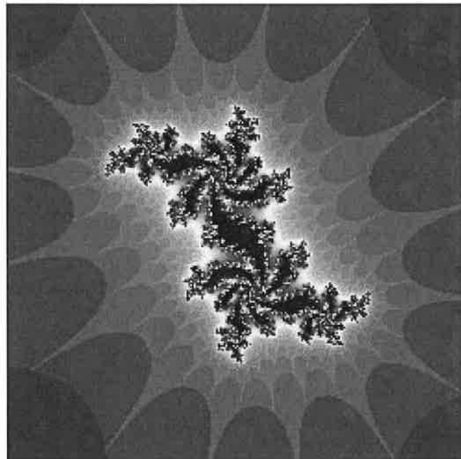
Conjunt de Julia f(z) = z^2 + 0,108+0,620i
