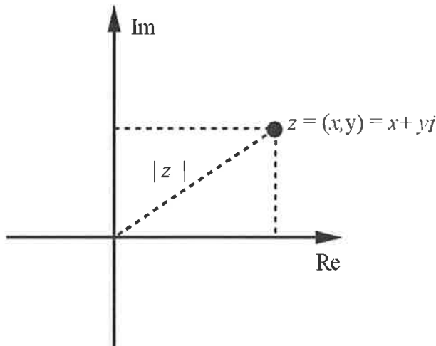
Nombre complex com a punt del pla complex
