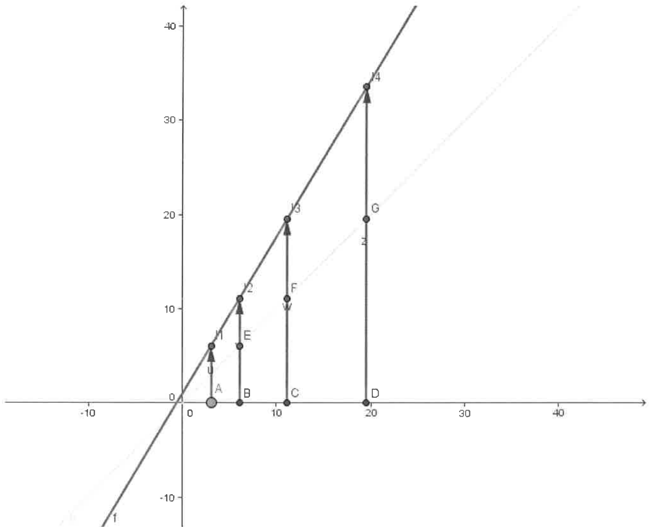
Gràfic de la funció f(x) = 5/3x + 1 , les seves quatre primeres iteracions i la funció Identitat
