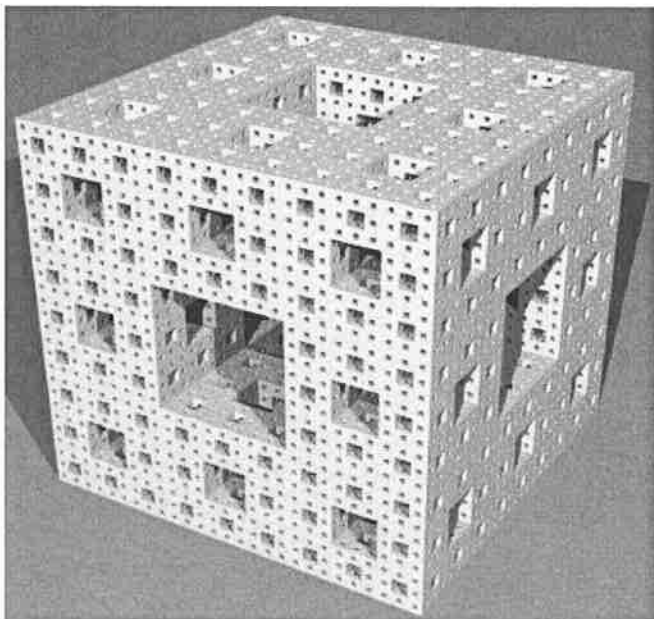
Esponja de Menger
