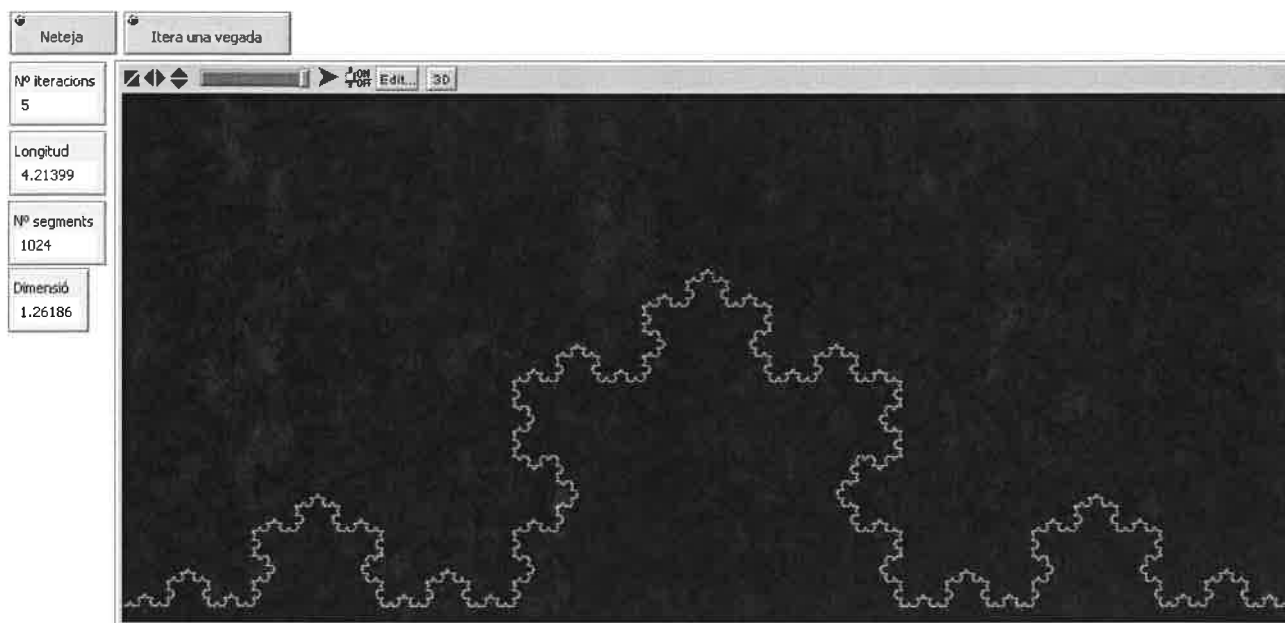
Corba de Koch dibuixada per NetLogo
