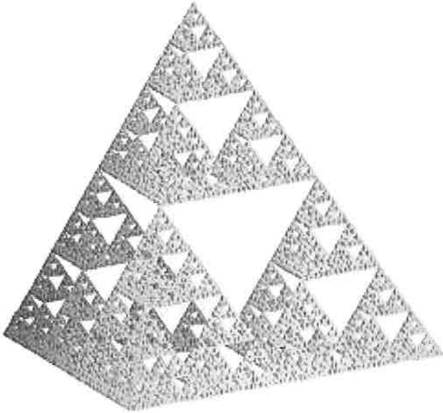
Tetraedre de Sierpiński
