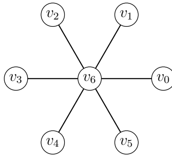
Figura 1.15: Graf estrella S_7
